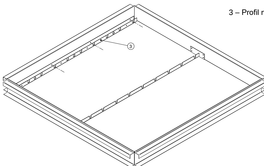
Rys. 28 Etap montażu profili nośnych kraty.
