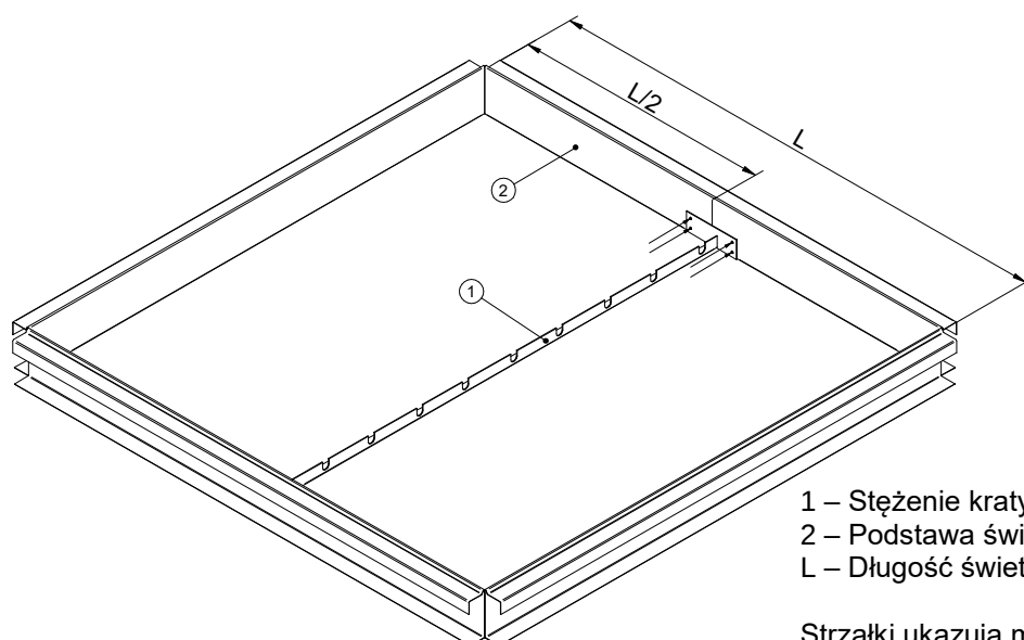
Rys. 27. Etap montażu stężenia kraty do podstawy świetlika.
