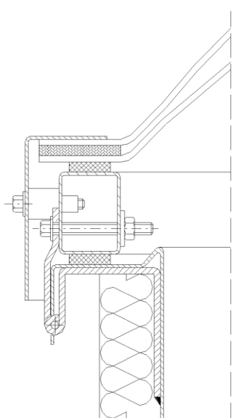
Rys. 2 Typowe wypełnienia świetlików i wyłazów mcr PROLIGHT.
