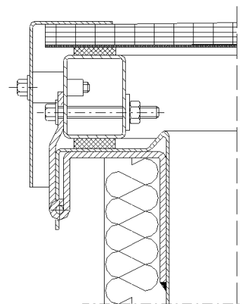
c) płyta poliwęglanowa i płyta poliestrowa (klasa B roof (t1))
